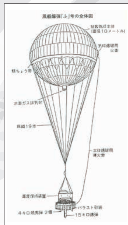
伴繁雄『陸軍登戸研究所の真実』 137頁より引用 (風船爆弾「ふ」号の全体図)
